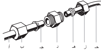
أ. أنابيب المياه الخاصة بالثلاجة ب. صامولة (مقدمة) ج. ماصباح د. وصلة (يتم شراؤها) هـ. حلقة وصل (يتم شراؤها) ز. صامولة (يتم شراؤها) ح. ماسورة المياه في المنزل
